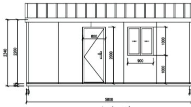
A elevation
