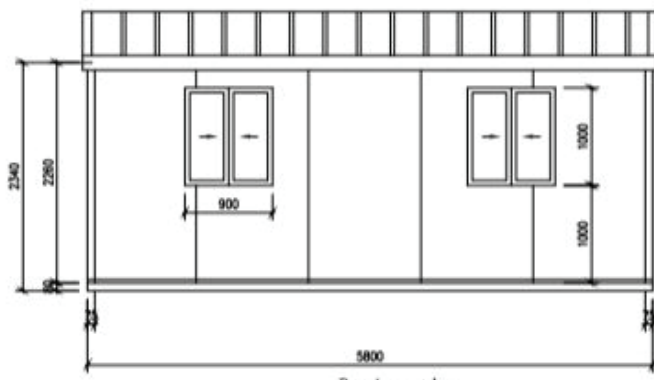
B elevation
